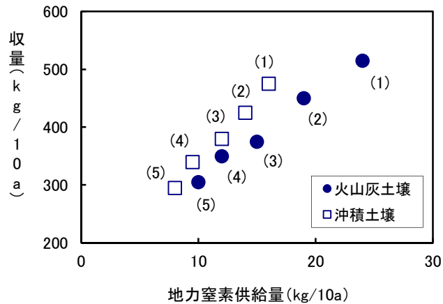
図3 転換畑での大豆作付け年数と地力窒素供給量及び収量の関係 (山形農試成績から作図)
